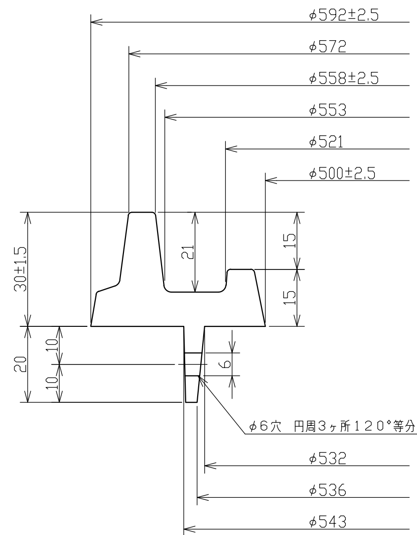
受枠断面詳細図 S = 1 / 1
