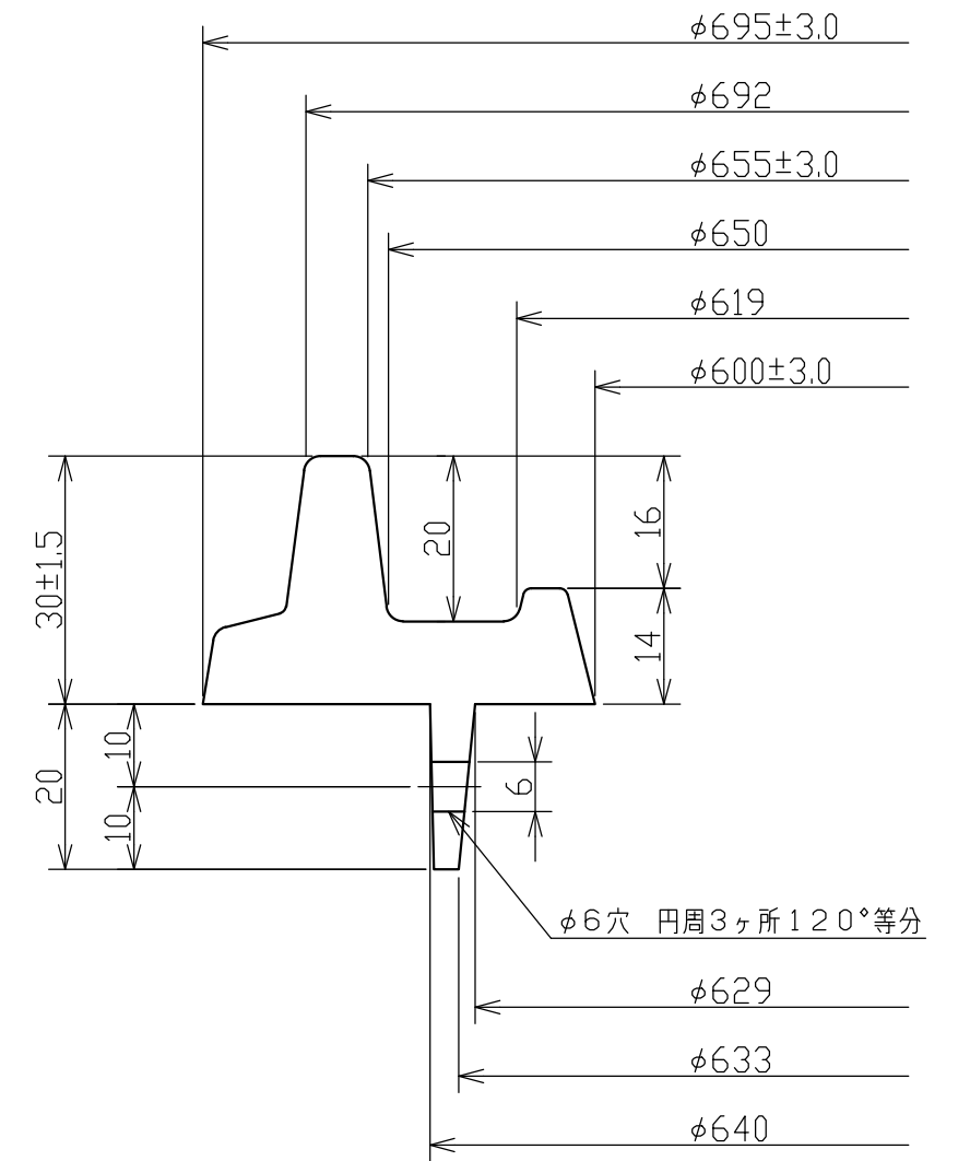
受枠断面詳細図 S = 1 / 1
