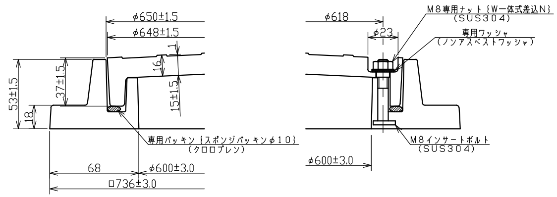
蓋・受枠・ロック部断面詳細図
