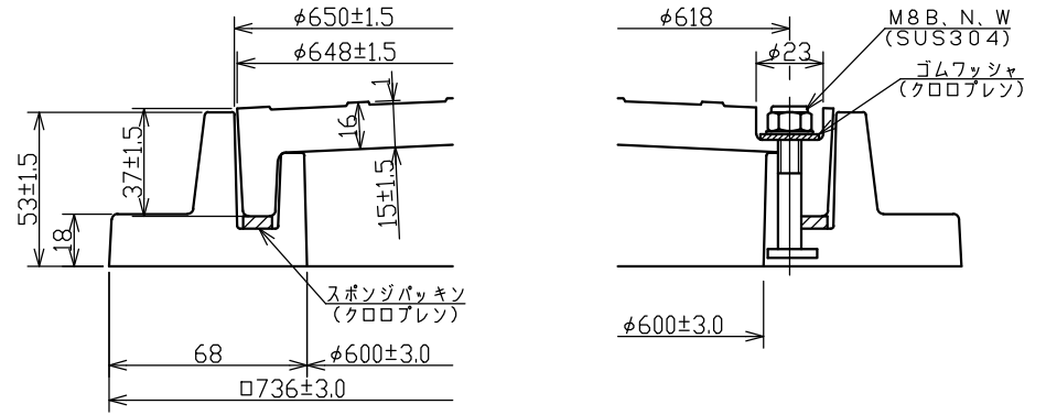
蓋・受枠・ロック部断面詳細図
