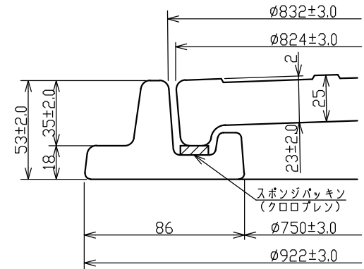
蓋・受枠断面詳細図
